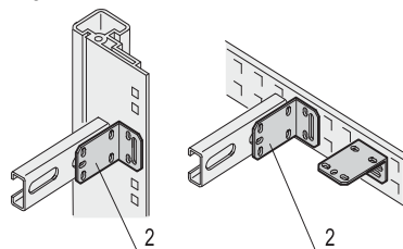
Универсальный кронштейн
