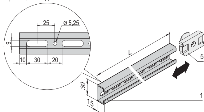
Монтажный кронштейн
