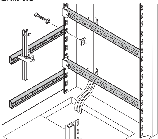
С-рельс/Закладная гайка
