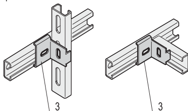
Универсальный кронштейн
