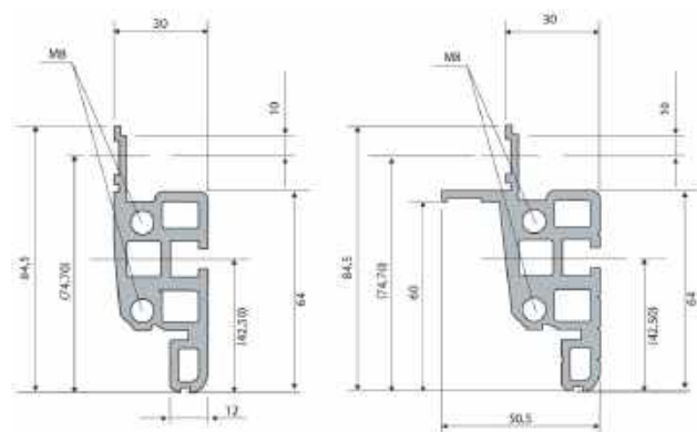
Универсальная стойка/19" задняя стойка
