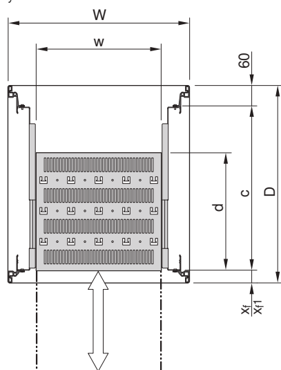
Укороченная глубина
