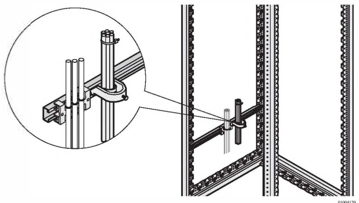
Планка крепления кабелей и кабельный зажим установлены на С-рельсе
