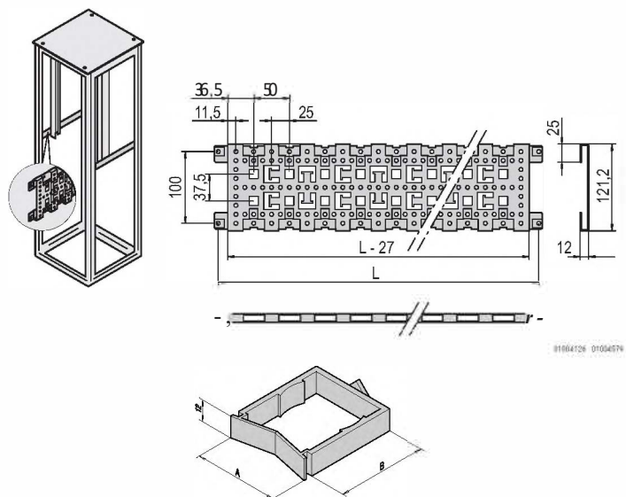
Кабельный органайзер
