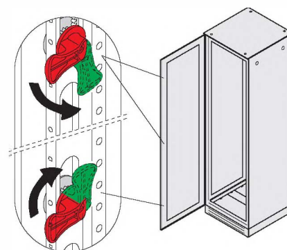
Трехточечная система запирания со встречными засовами
