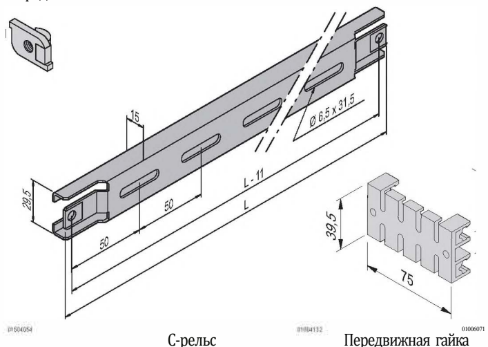
Передвижная гайка
