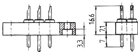
Размерный эскиз штекерной части разъема
