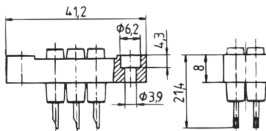
Размерный эскиз штекерной части разъема
